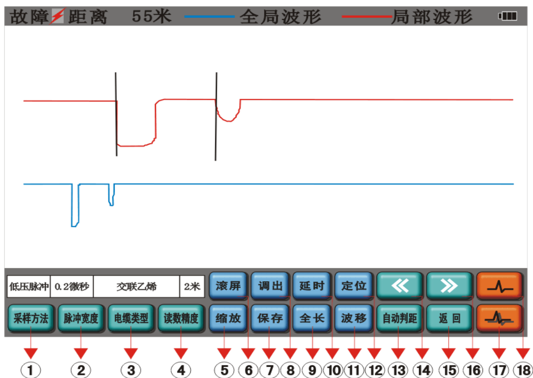
图三 液晶屏菜单显示示意图
